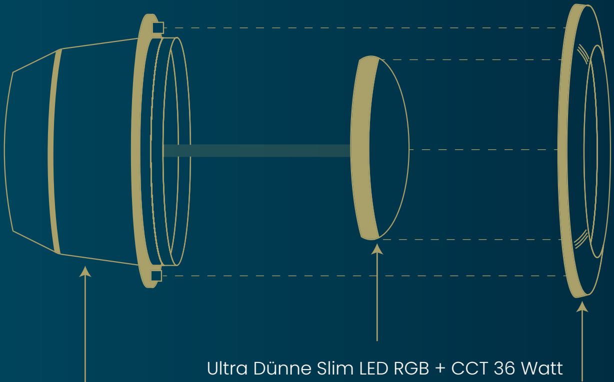
PAR56 Universal Einbautopf
